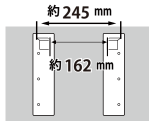
背面フック寸法
