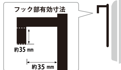
フック詳細
