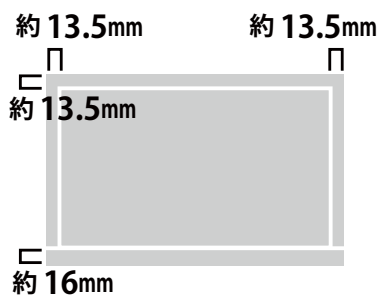
ディスプレイ箱寸法図
