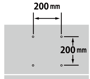
背面寸法
