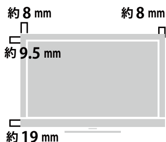
ベゼル寸法
