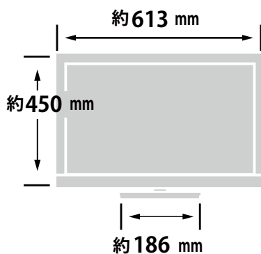
ベゼル寸法
