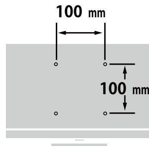
背面寸法
