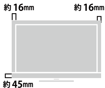
ベゼル寸法
