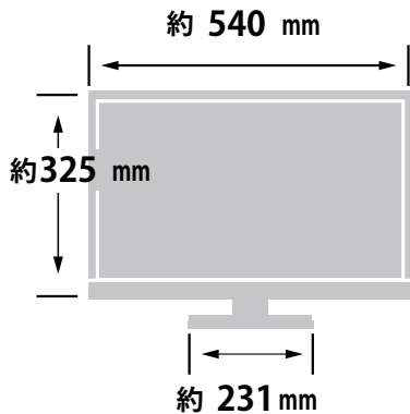
外形寸法
