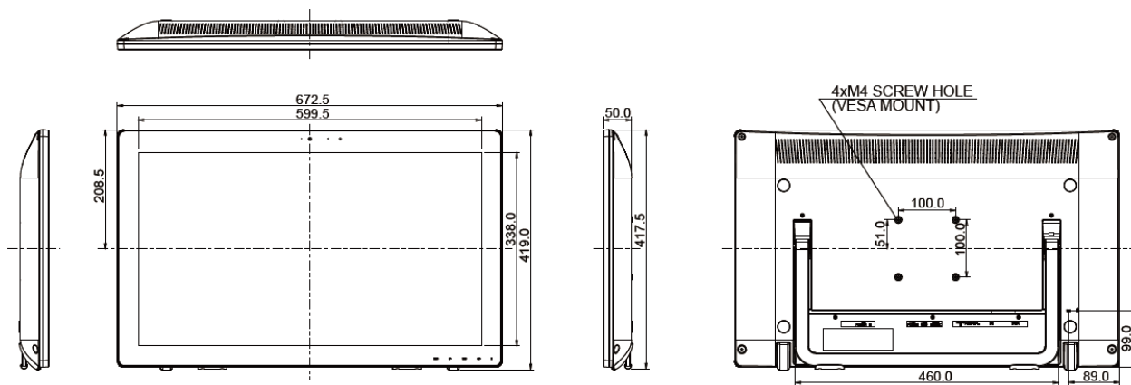
寸法図
